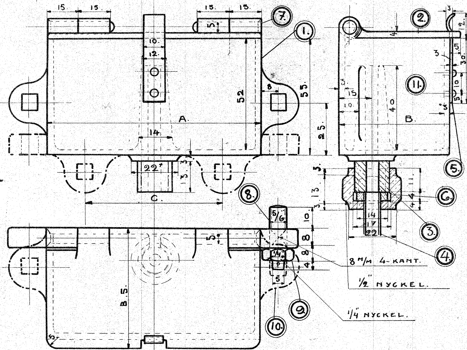
SMÖRJKOPP MED ÖRON ENL. = A. " " " " = B. " " " " = C.
